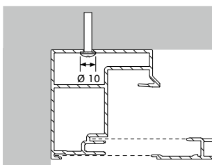
Montage achterwand zijgeleider Fixscreen® Mono AK
