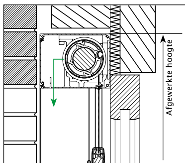
Voorbouw, voor/boven het raam met kast
