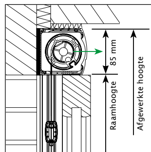
Opbouw, bovenop het raam met omgekeerde kast, zonder voorkap
