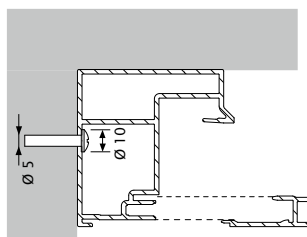
Zijdelingse montage zijgeleider Fixscreen® Mono AK
