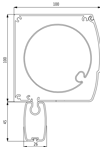
Geleiders voor Fixscreen® 100 EVO & 150 EVO
