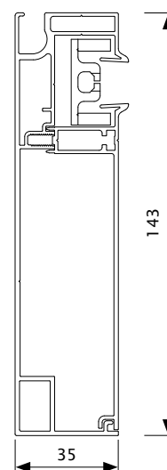
diepe zijgeleider (D)
