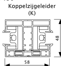
Geleiders voor Fixscreen® 100 EVO & 150 EVO
