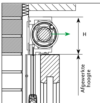
Inbouw, met beugels, zonder kast
