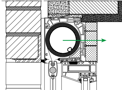
Montagesituatie 4: Fixscreen® Mono AK Medium+
