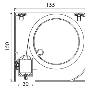
Fixscreen® 150 EVO / Fixscreen® 150 EVO F
