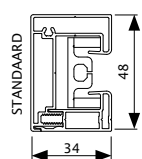
Zijgeleider (S)
