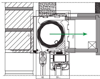
Montagesituatie 4: Fixscreen Mono AK - afwerking schrijnwerker
