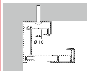
Montage achterwand zijgeleider Fixscreen® 85
