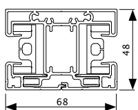
Koppelzijgeleider (K)
