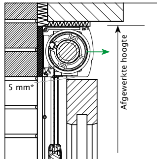
Opbouw, bovenop het raam met omgekeerde kast, zonder voorkap * 5 mm extra voorzien tussen raamhoogte en onderzijde Fixscreen*
