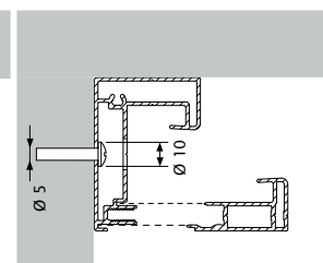
Zijdewandse montage zijgeleider Fixscreen® 85
