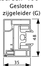
Geleiders voor Fixscreen® 100 EVO & 150 EVO
