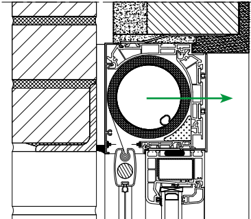
Montagesituatie 4: Fixscreen® Mono AK Small
