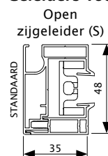
Geleiders voor Fixscreen® 100 EVO & 150 EVO
