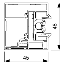
standaard zijgeleider (S)
