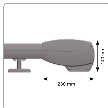
Afmetingen kast
